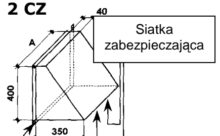
2 CZ Czerpnia powietrza Kołnierze 25 mm z 4 stron
