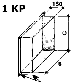
1 KP Kołnierze 25 mm z 4 stron
