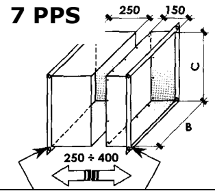
7 PPS Przejście teleskopowe przez ścianę Kołnierze 25 mm po 2 stronach
