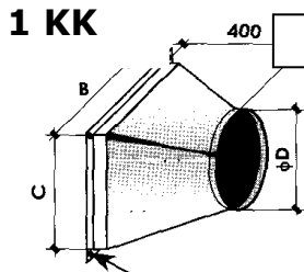
1 KK Kołnierze 25 mm z 4 stron
